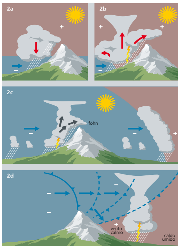
Fig. 26 Il fronte freddo sale lungo la catena montuosa e la valica. 2a-b) spessore dell'aria fredda minore della catena montuosa: caso stabile (a) e instabile (b), in entrambi le precipitazioni rimangono da un lato della catena 2c) spessore maggiore, forte vento in quota: precipitazioni da una parte della catena montuosa, dall'altra foehn 2d) spessore maggiore, vento debole in quota: precipitazioni da una parte della catena montuosa, forte instabilità dall'altra
