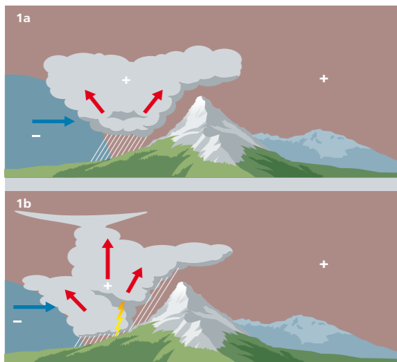
Fig. 25-26 Schema dell'interazione di un fronte freddo con le Alpi
